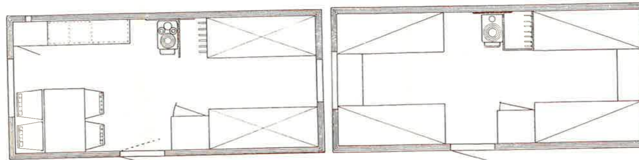
A2 Sovebrakke med 4 køyer.
